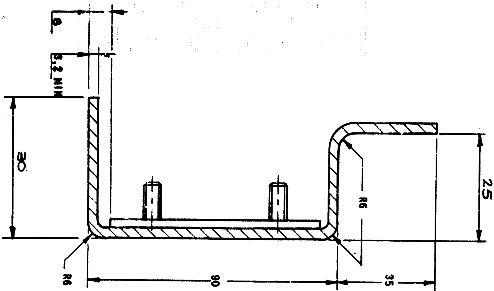
SECTION Y-Y SCALE: 1:1
