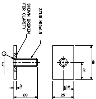
ITEM 4 - DRG No 264888 & ITEM 5 DRG 264891
